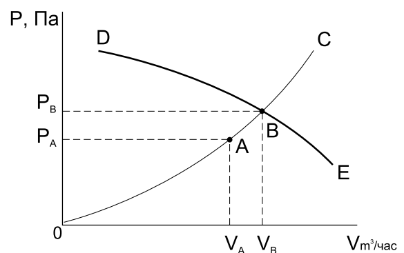
Рис. 3. Пересечение характеристики сети О-А-В-С с характеристикой вентилятора DE.
