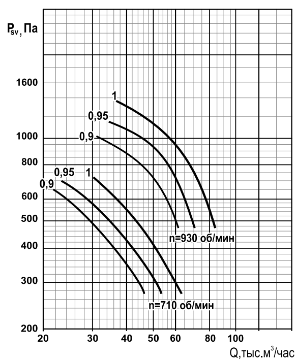
ВКР1ДУ-12,5 ВКР2ДУ-12,5
